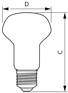
R63 220-240V 7W 650lm 2700K E27 ND
